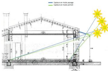
Simulation sur photo et schéma du brise-soleil de Gaubert
